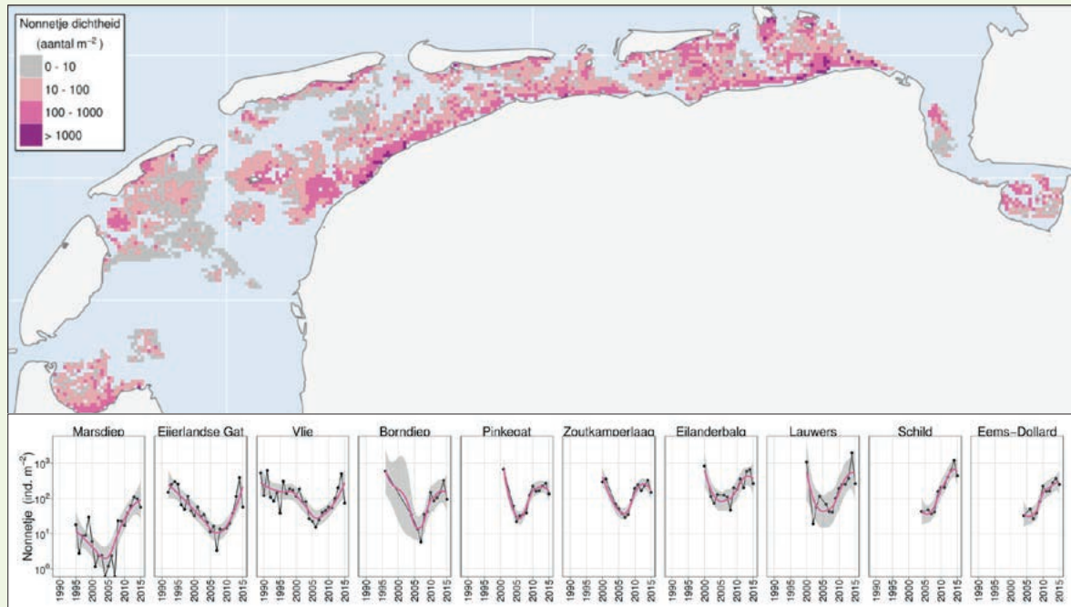
Figuur 3 (a) Verspreiding van en (b) trends in dichtheden van Nonnetjes (aantallen schelpdieren per m 2 ) vanaf 2008 t/m 2015 (Data: NIOZ/SIBES)
