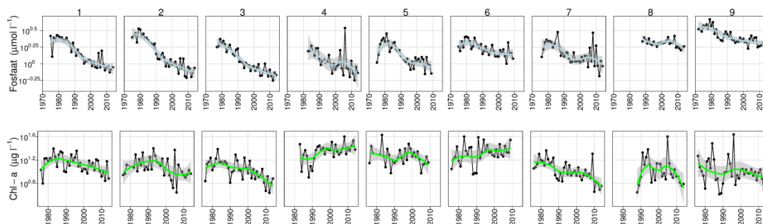
Figuur 2 Verloop in concentraties van fosfaat ( \mu\text{mol PO}_4^{2-} per liter) en dichtheden van fytoplankton ( \mu\text{g} chlorofyl-a per liter) in het zeewater van 1976 t/m 2014 (Data: Rijkswaterstaat)
